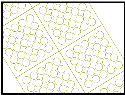
SV03 SOLADO DE VEREDA LOSETA PODOTACTIL
